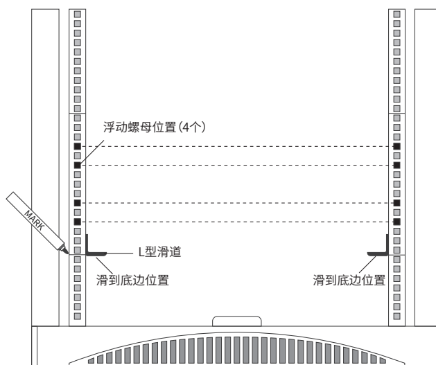
图2-2 标记浮动螺母和L型滑道位置
